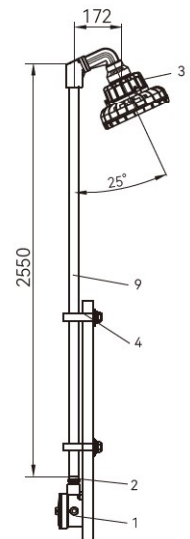
护栏式(h2)
