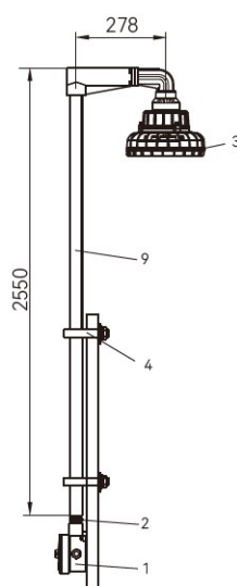
护栏式(h1)
