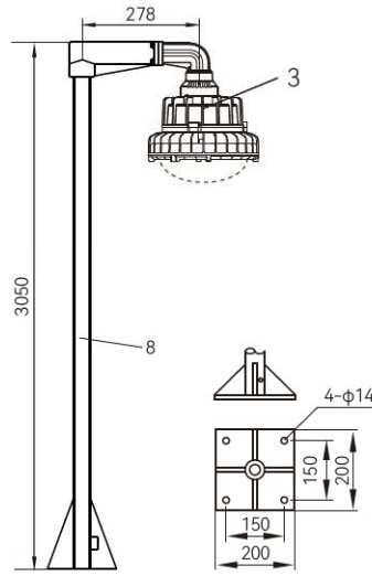
法兰式(F1)
