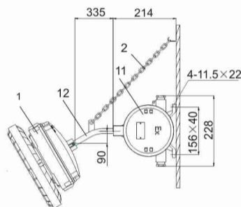
配应急,壁式(B1)30°
