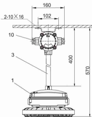
配吊灯盒杆子
