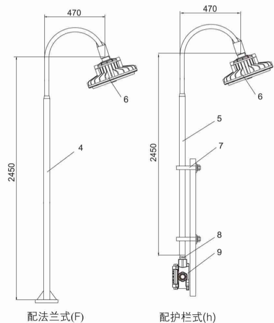
配吊灯盒杆子
