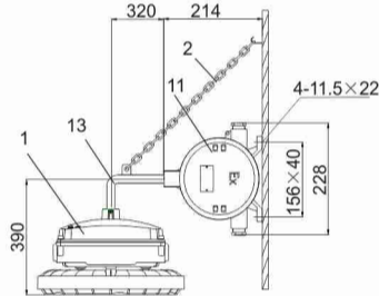
配应急,壁式(B2)90°
