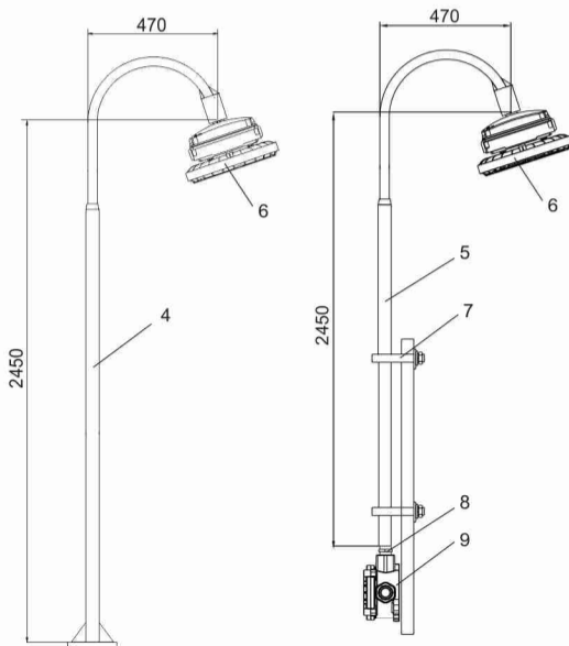
配法兰式(F)
