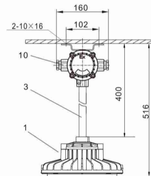
配吊灯盒杆子
