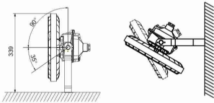
吸顶式(支架式)(X)
